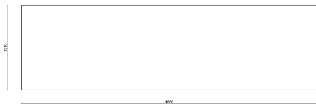
LAMIERA Zn - \frac{10}{10} - FISCHERATA CON TASSELLI IDONEI PER ESTERNO
